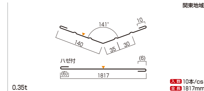
谷板(小)リップ35/65ハゼ付 品番 Y-535H 関東地域
