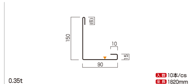
L型捨板 品番 Y-570
