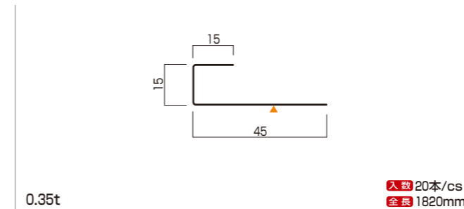
■ 広小舞キャップ 15×15×45 品番 Y-150
