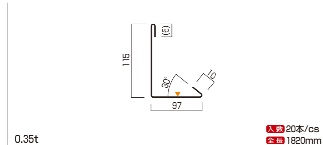
洋瓦用捨板 品番 Y-561
