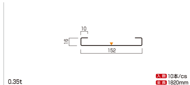
平板瓦用捨板継ぎ 品番 Y-564
