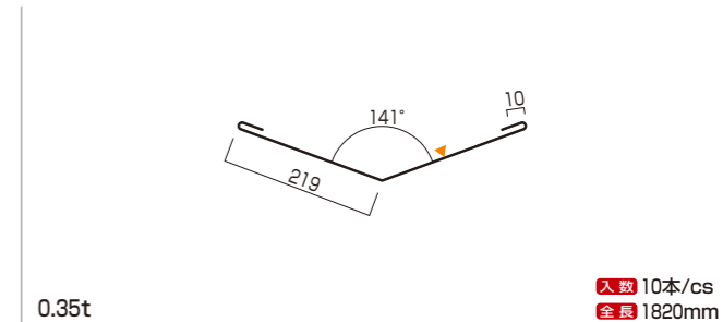
洋瓦用谷板 品番 Y-560
