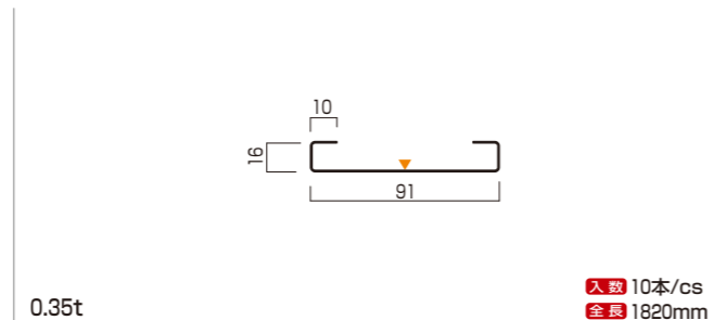
ケラバ捨水切 品番 Y-565
