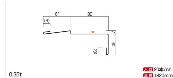
■ 雪国用軒先水切 品番 Y-120
