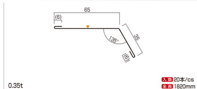
■ 軒先水切 35×65(135°) 品番 Y-108
