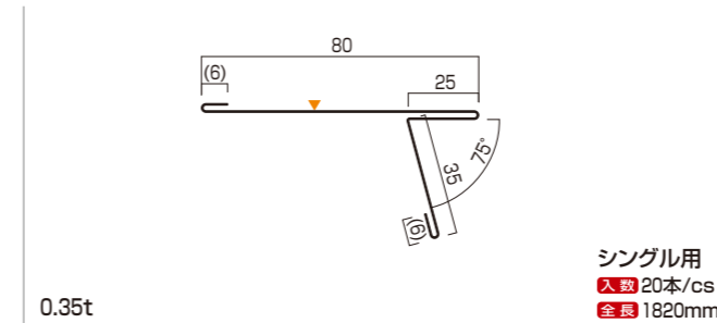
■ 重ね葺き用軒先水切 品番 YS-118
