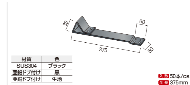
雪止め金具 品番 Y-901
