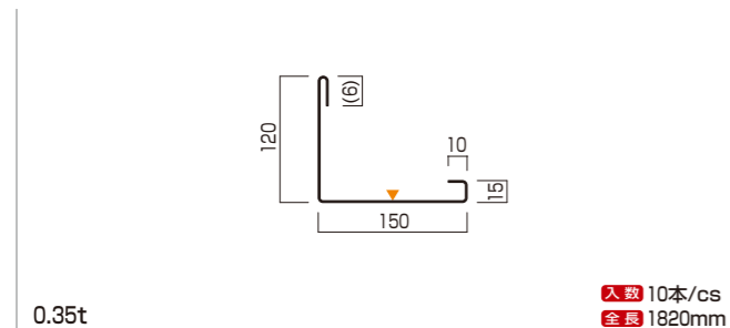
平板瓦用捨板 品番 Y-563
