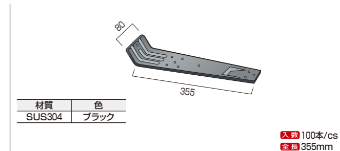
雪止め金具(後付け用) 品番 Y-902
