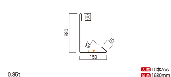
L型捨板(大) 品番 Y-571
