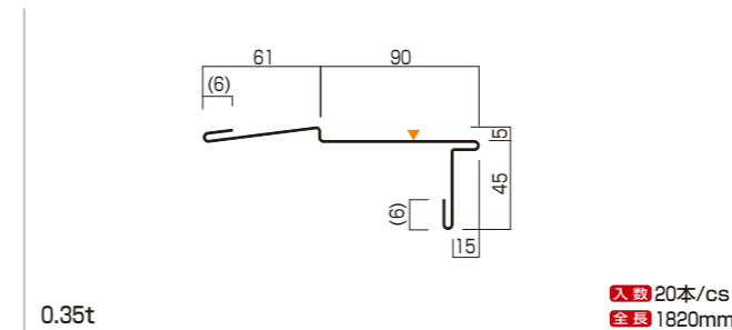
■ 雪国用軒先水切(ツノ付き) 品番 Y-121
