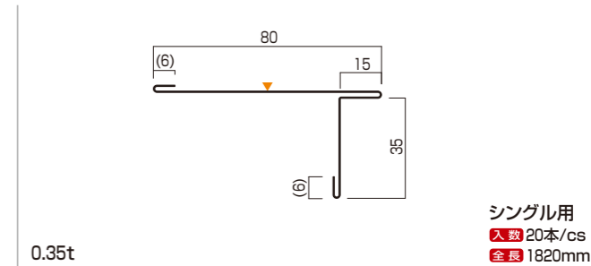
■ 軒先唐草 T 品番 YS-115
